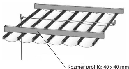
Rozměr profilů: 40 x 40 mm
