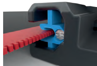
Detail vodící kolejkice se zipem
